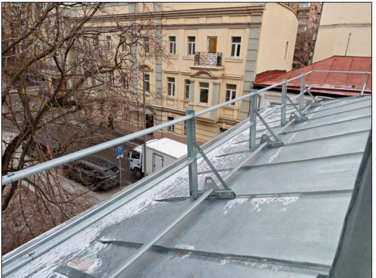
Фото 8. Общий вид кровельного ограждения.
