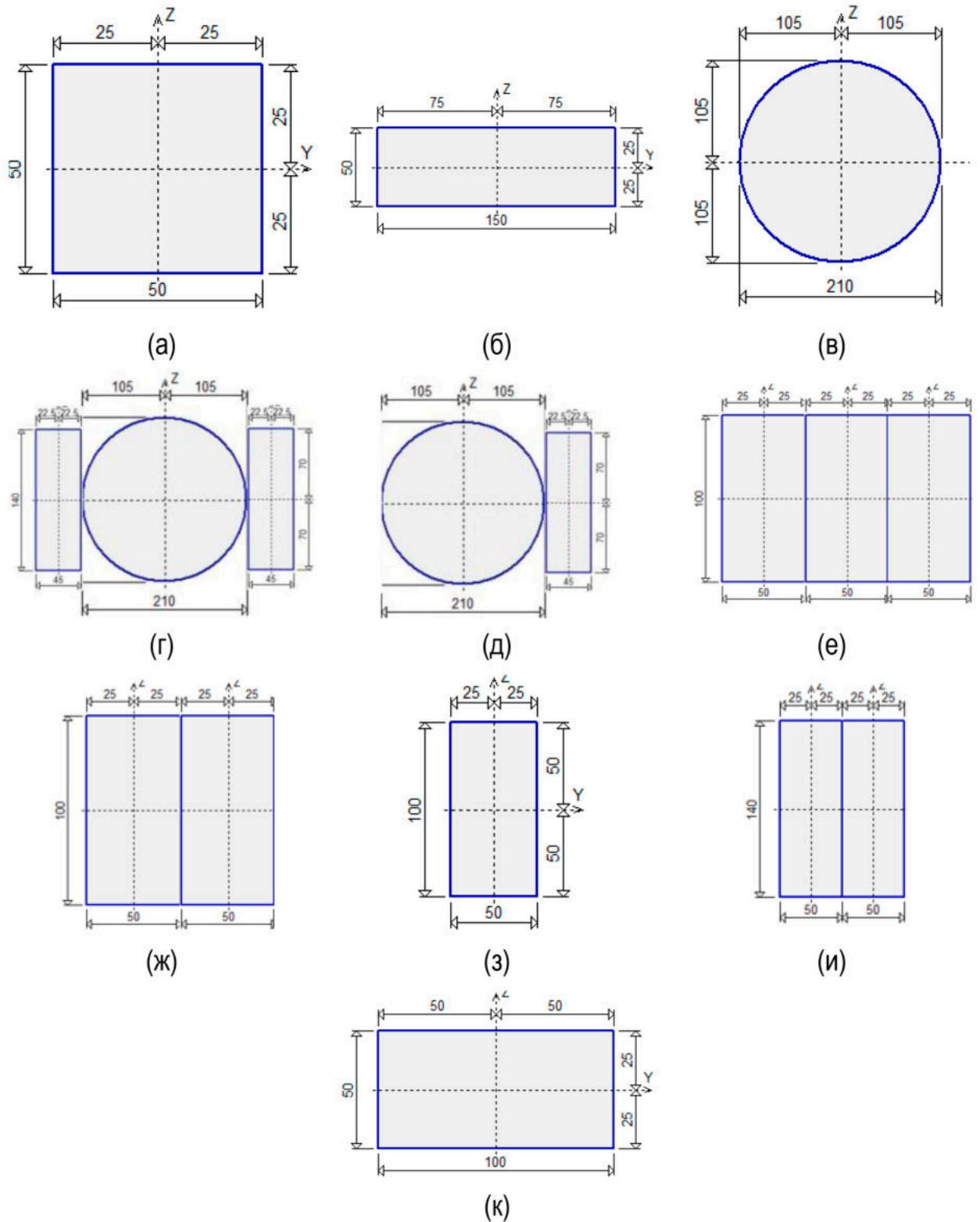
Рис.3 Характерные сечения элементов конструкций крыши, где а – сечение контробрешетки, б – сечение обрешетки, в – сечение стропильной ноги и мауэрлата, г – сечение стропильных ног С1, д – сечение стропильных ног С2, е – сечение стропильных ног С4, ж – сечения стропильных ног С3, з – сечение затяжки, и – сечение стойки, к – сечение лежня.
