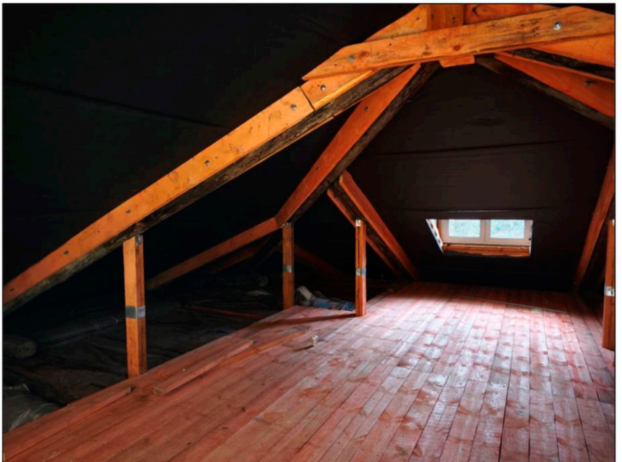
Фото 2. Общий вид стропильных конструкций Объекта экспертизы.
