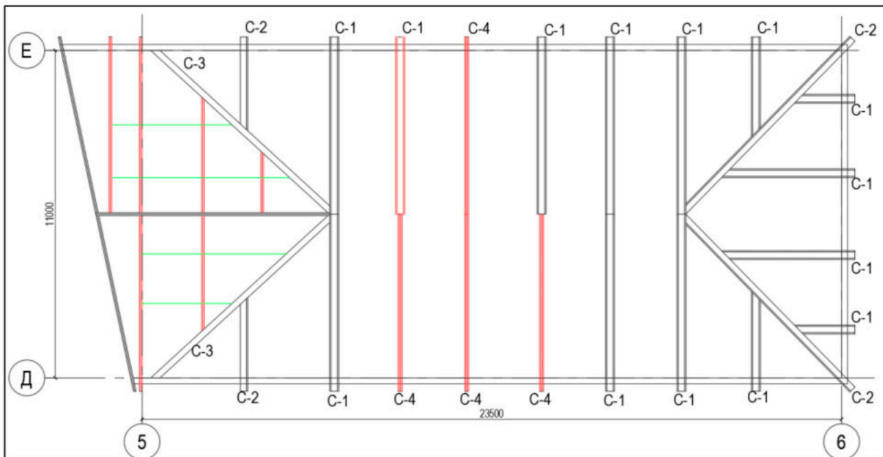
Рис.4 План стропил с расположением характерных элементов, где красным выделены стропила, которые необходимо усилить; зеленым выделены прогоны, которые необходимо добавить.
