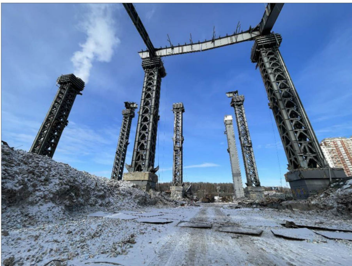
Фото 2. Частный вид Объекта в осях «А-Н/33-35».
